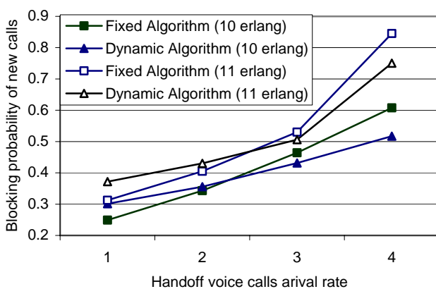
شکل ۴: تغییرات احتمال رد درخواستهای جدید در روش پویای پیشنهادی و روش ثابت نسبت به افزایش نرخ ورود درخواستهای تحویل کانال سرویس صوت (در بار ترافیکی ثابت ۱۰ و ۱۱ ارلنگ)
