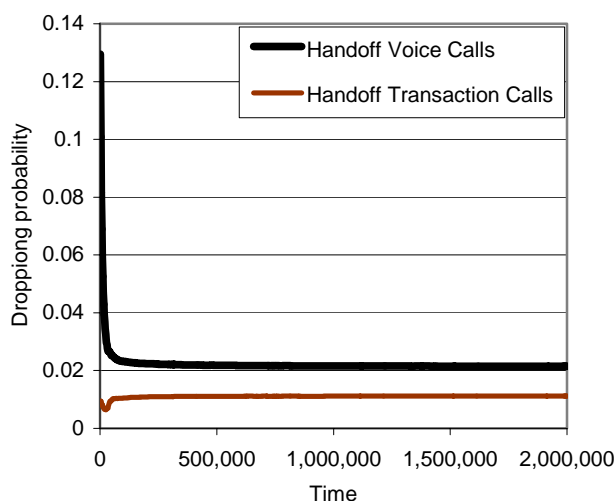
شکل ۶: همگرایی احتمال قطع درخواستهای تحویل کانال سرویسی صوت و تراکنش با استفاده از الگوریتم پیشنهادی
