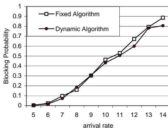
شکل ۵: احتمال رد درخواستهای جدید کانال با استفاده از الگوریتم پیشنهادی و الگوریتم ثابت
